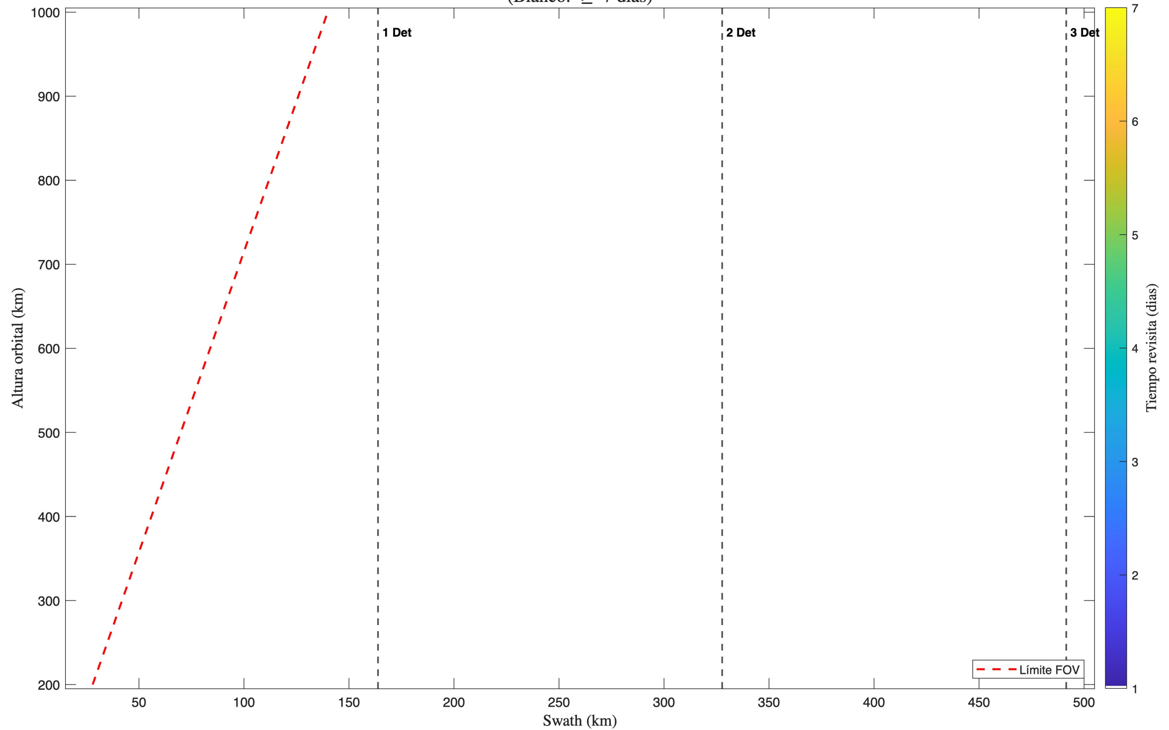
Tiempo Revisita - 2 Satelite(s); 1 Telescopio(s): TMA; Detector 2 (Blanco: \geq 7 dias)
